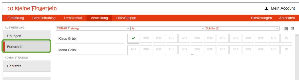
Abbildung 7: Übungsfortschritt
