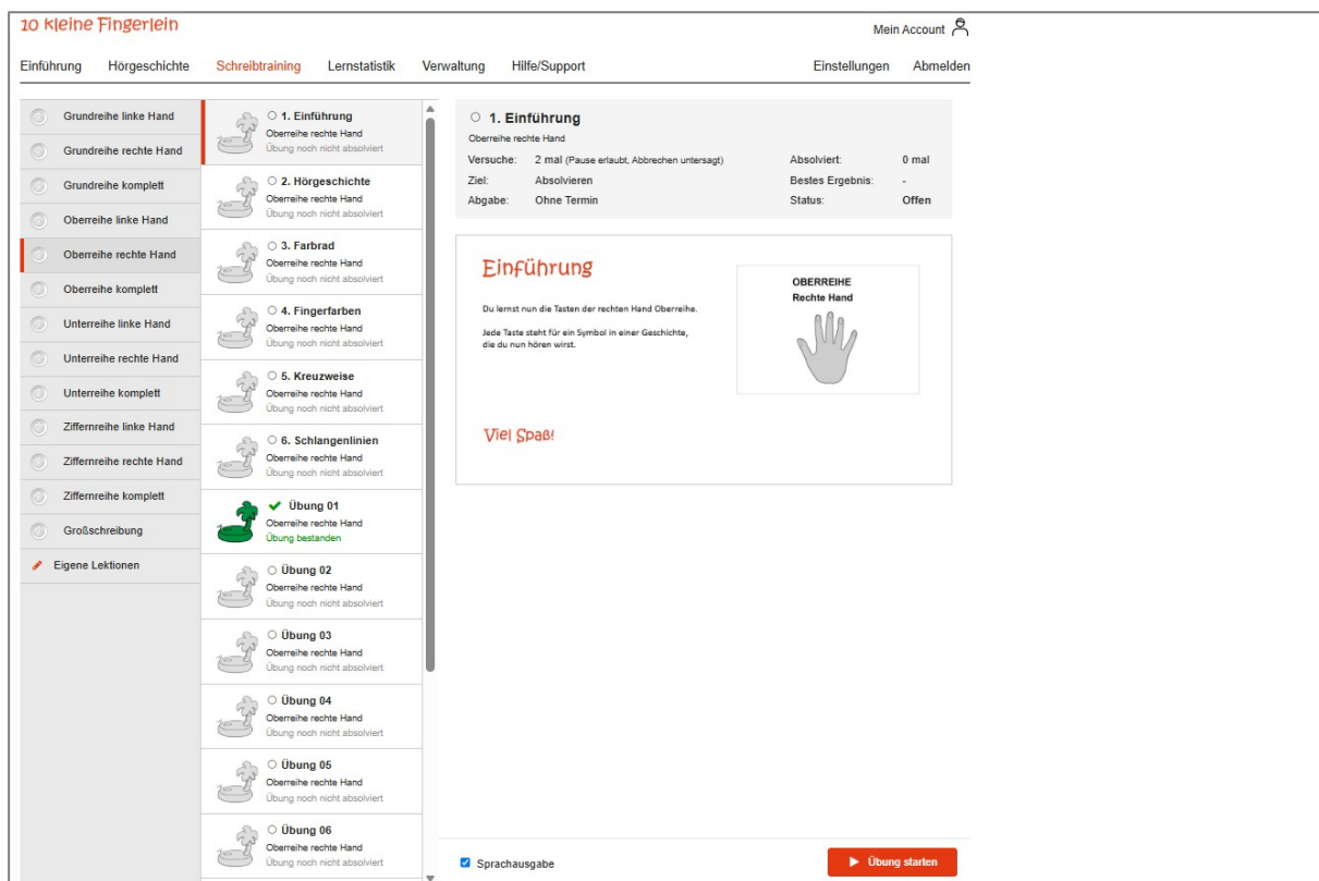
Abbildung 6: Oberfläche Schreibtraining
