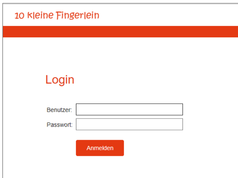
Abbildung 3: Login-Seite
